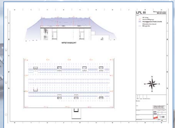
Planta fotovoltaica
